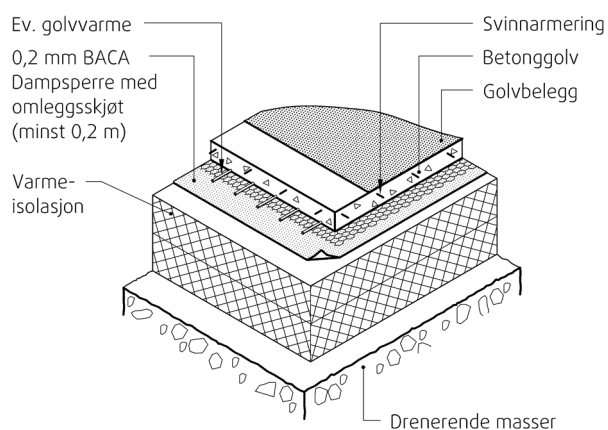
Fig 3 BACA Dampspærre montert i betonggulv på grunnen
